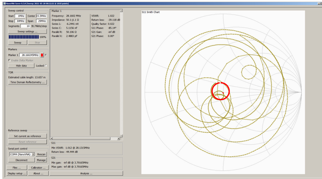
Bild 14: Smith Chart der EndFed-Antenne
