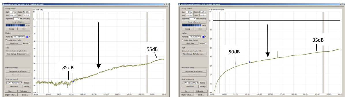
Bild 9: Grenzen der Übertragungs- (links) und S11 Rückflußdämpfung(rechts)
