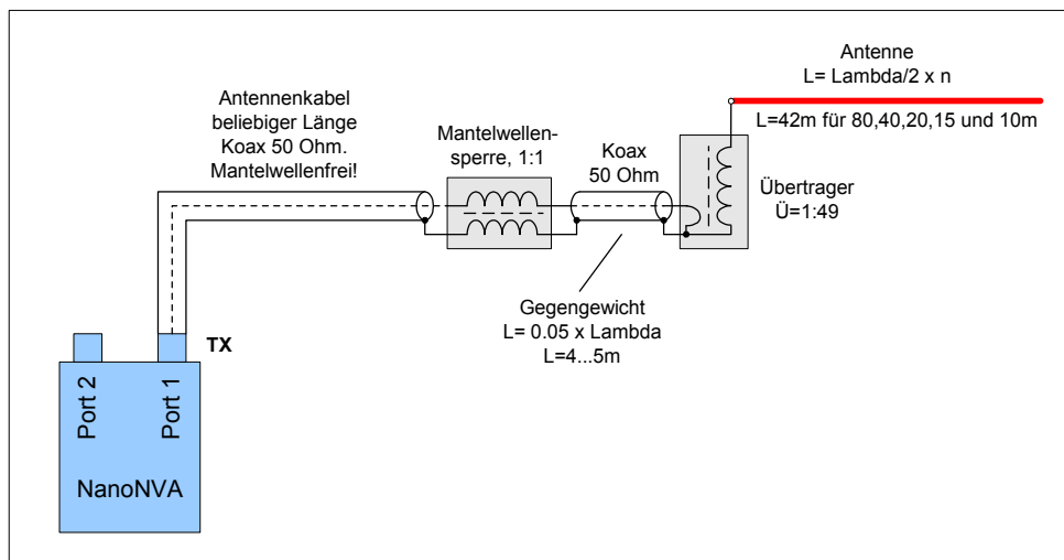
Bild 10: Aufbau und Verbindung der EndFed-Antenne an den NanoVNA, Port1, S11
