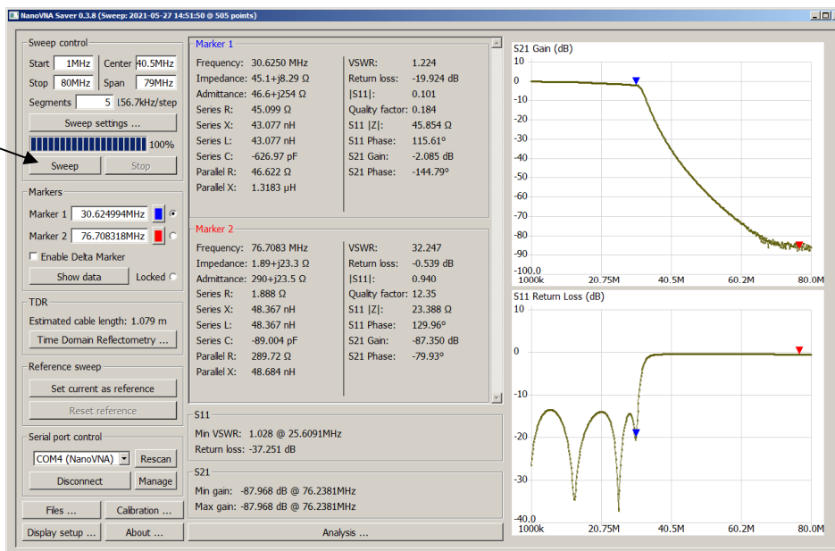
Bild 7: Messung von Übertragung S21 und Rückflußdämpfung S11 des TP-Filters am PC
