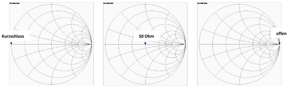
Bild 1: Prüfung der Kalibration mit Hilfe der Smith Chart
