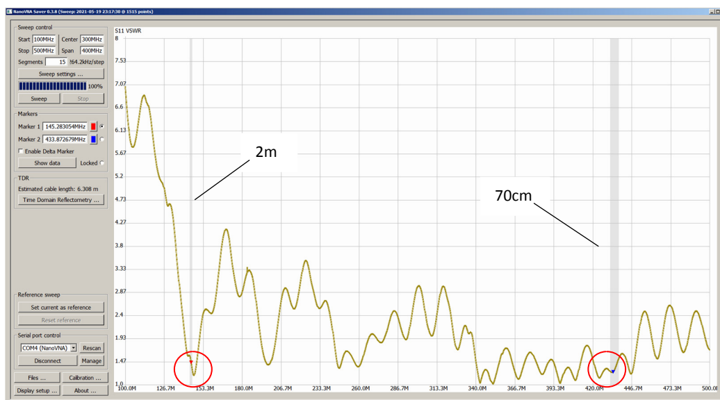
Bild 15: VSWR-Verlauf einer 2m/70cm-Antenne
