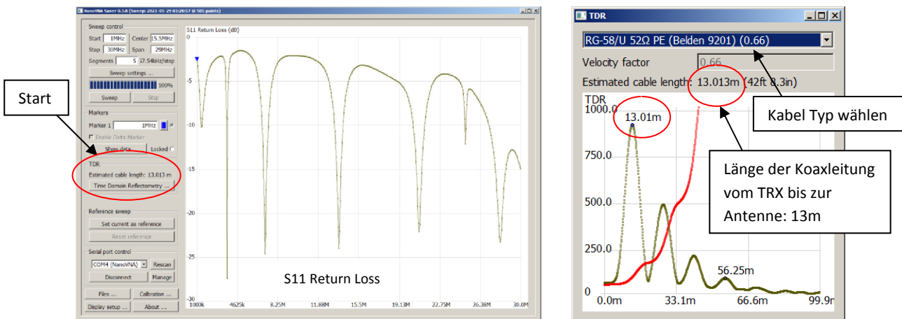
Bild 21: TDR-Messung am Antennenkabel
