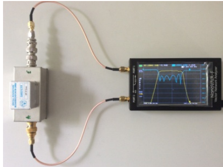
Bild 18: Messung an einem Quarzfilter
