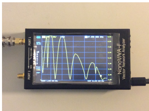
Bild 11: VSWR-Kurve meiner Antenne am NanoVNA
