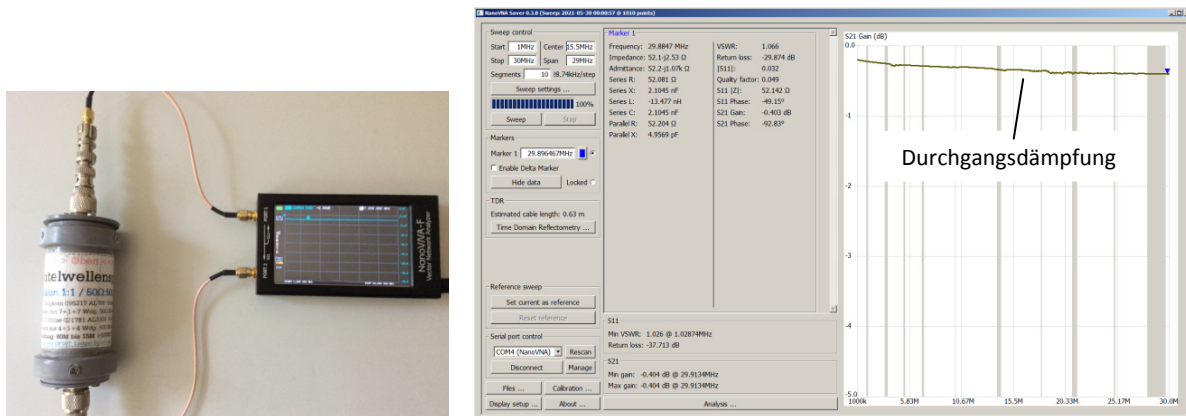
Bild 17: Durchgangsdämpfung der Mantelwellensperre
