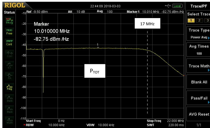
Bild 7: Rauschkurve bis 17MHz, Rauschleistung -83dBm/Hz, P_{TOT} = -10,7\text{dBm/17MHz}
