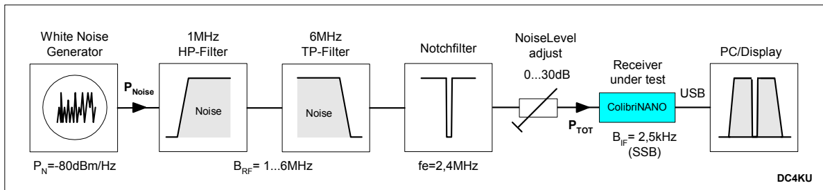
Bild 1: NPR (Noise Power Ratio) - Messplatz
