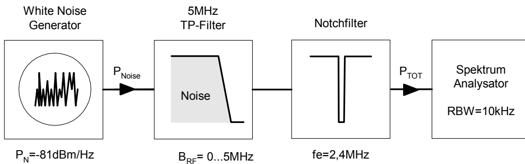
Bild 4: Schaltung für NPR-Messung mit 5MHz TP-Filter und 2,4MHz Notchfilter
