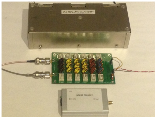
Bild 8: Rauschgenerator, wählbare TP-Filter und Notch-Filter
