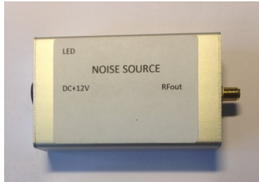
Bild 1: Rauschgenerator mit einer eingestellten Rauschleistung von -81dBm/Hz und flacher Rauschkurve
