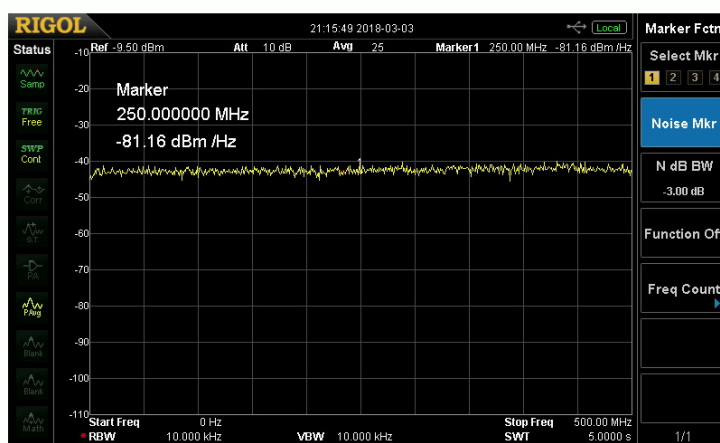
Bild 3: Verlauf der Rauschkurve von 0 bis 500MHz, Rauschleistung = -81dBm/Hz, RBW 10kHz
