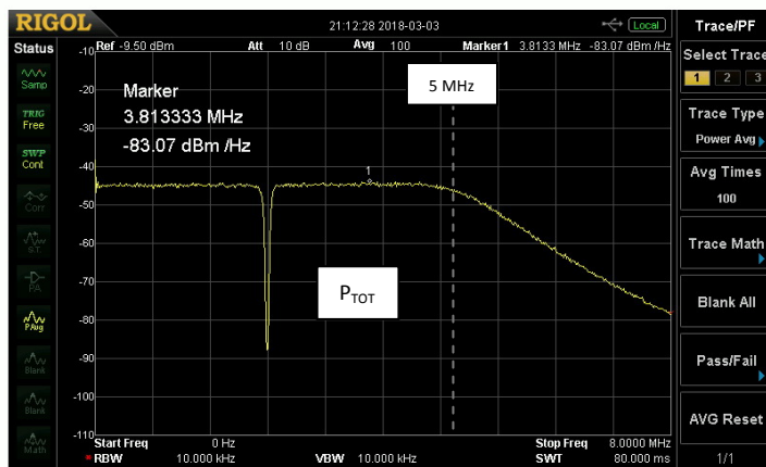
Bild 5: Rauschkurve mit Notch- und TP-Filter, Rauschleistung -83dBm/Hz, P TOT = -16dBm/5MHz
