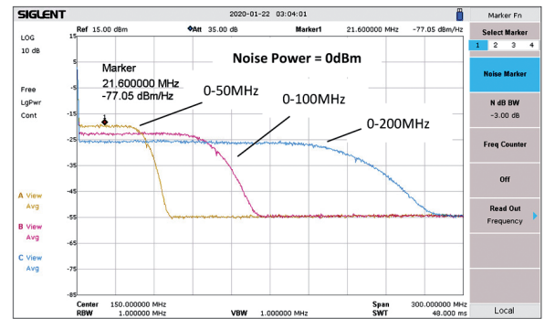
Bild 2: Rauschsignale des SDG6022X
