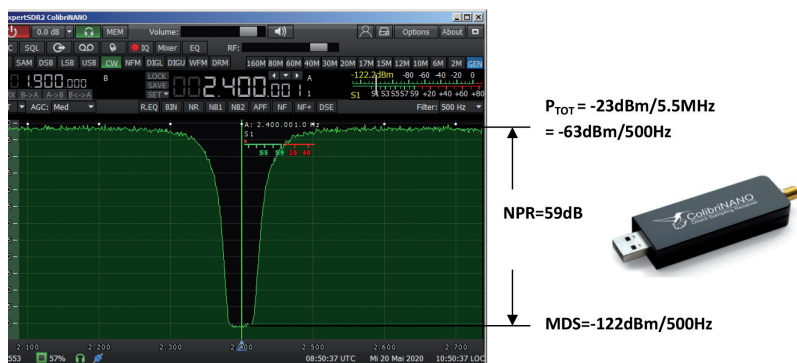
Bild 6: ColibriNANO mit BRF = 5,5 MHz, NPR = 59 dB
