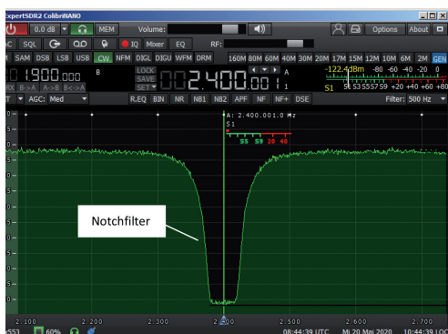
Bild 5: ColibriNANO mit BRF = 55 MHz, NPR = 49 dB
