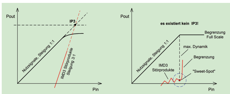
Bild 1: Prinzipieller IMD3-Verlauf eines analogen (links) und eines digitalen Empfängers (rechts)
