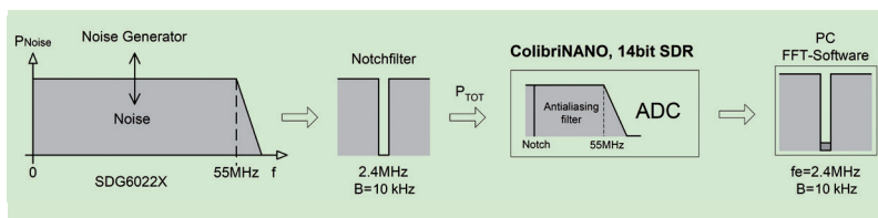
Bild 4: NPR-Messung am ColibriNANO
