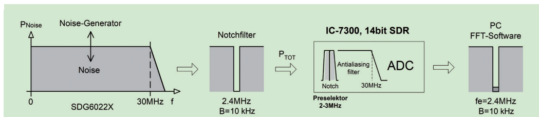
Bild 8 (unten): NPR-Messung am IC-7300
