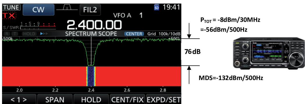
Bild 9: IC-7300, NPR = 76 dB
